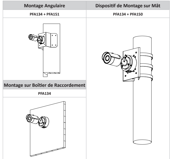
PFA134 Boîte de Raccordement
