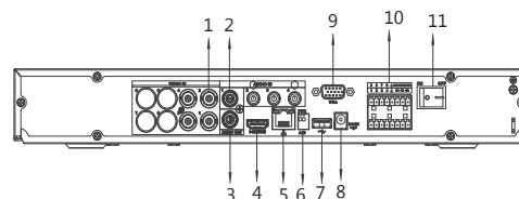
DHI-XVR5204A-S2
