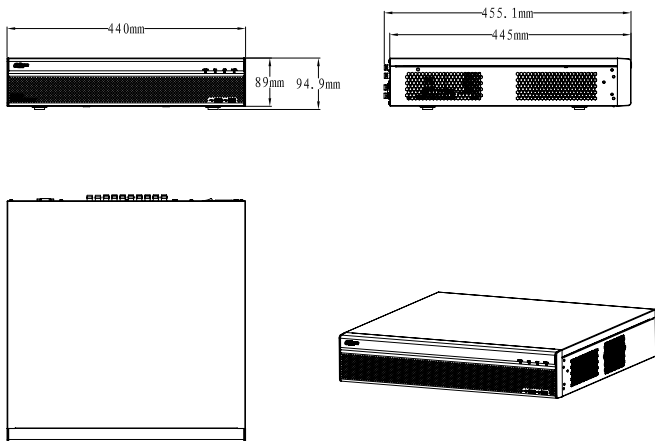
DHI-XVR5832S
