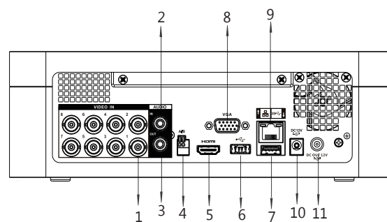
DH-XVR7108E-4KL-B-X
