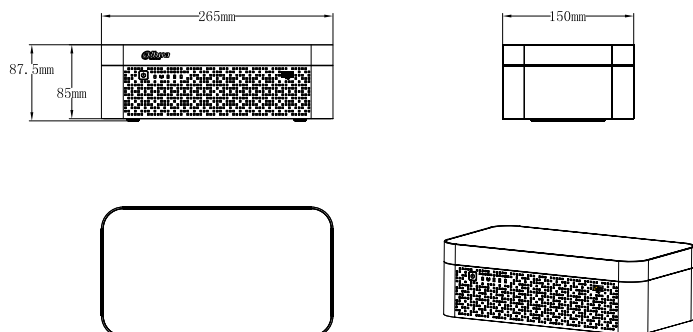
DH-XVR7108E-4KL-B-X
