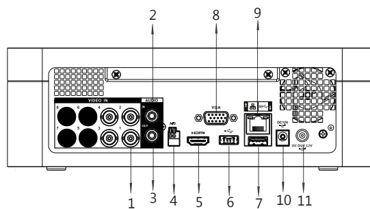
DH-XVR7108E-4KL-B-X
